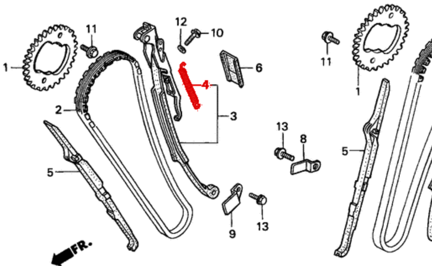
Schemat: Honda XL600V Transalp PD10
